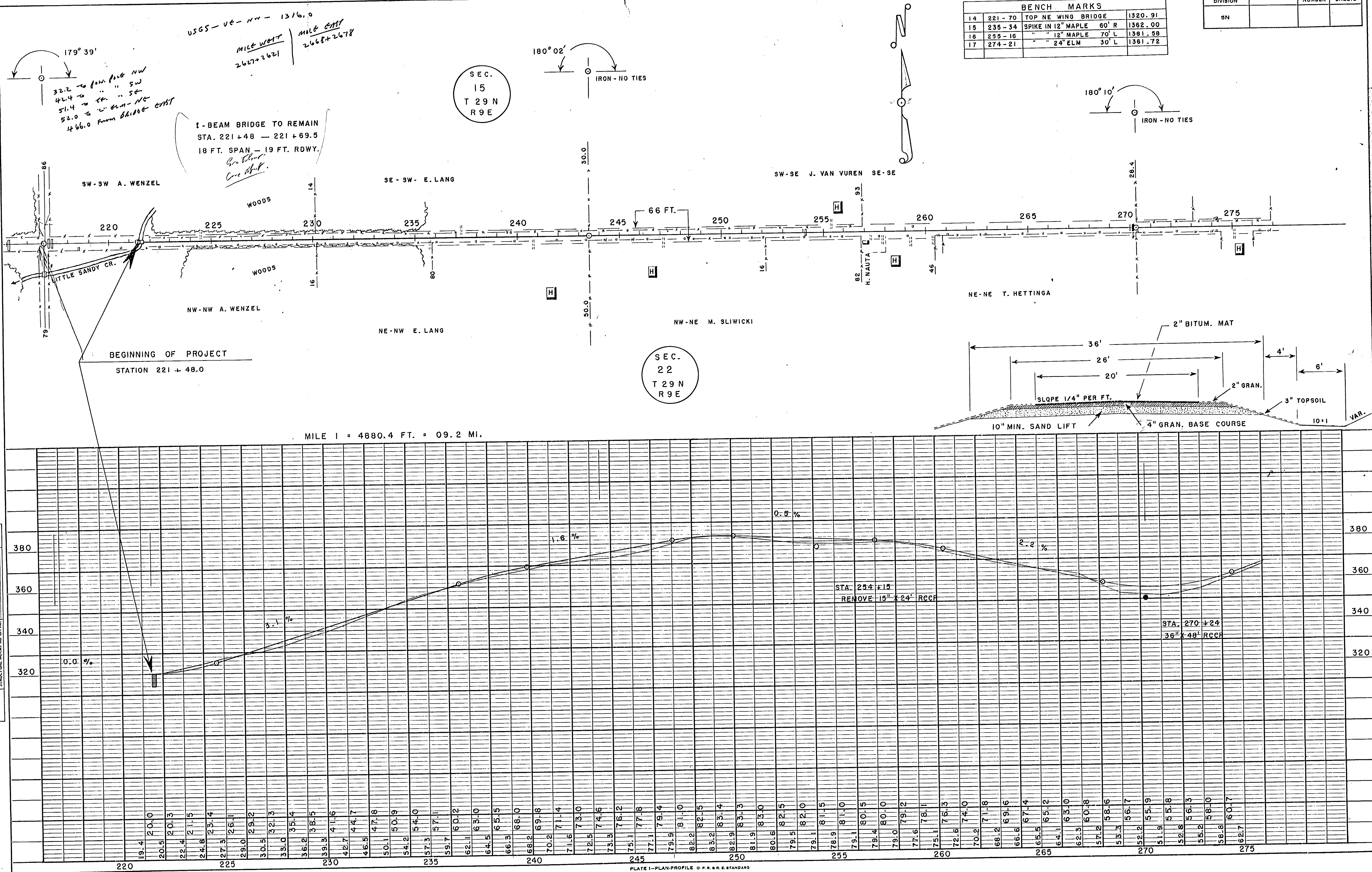
PLATE 1-PLAN-PROFILE O. P. R. & R. E. STANDARD THE HOLLISTON MILLS, INC. CHICAGO
